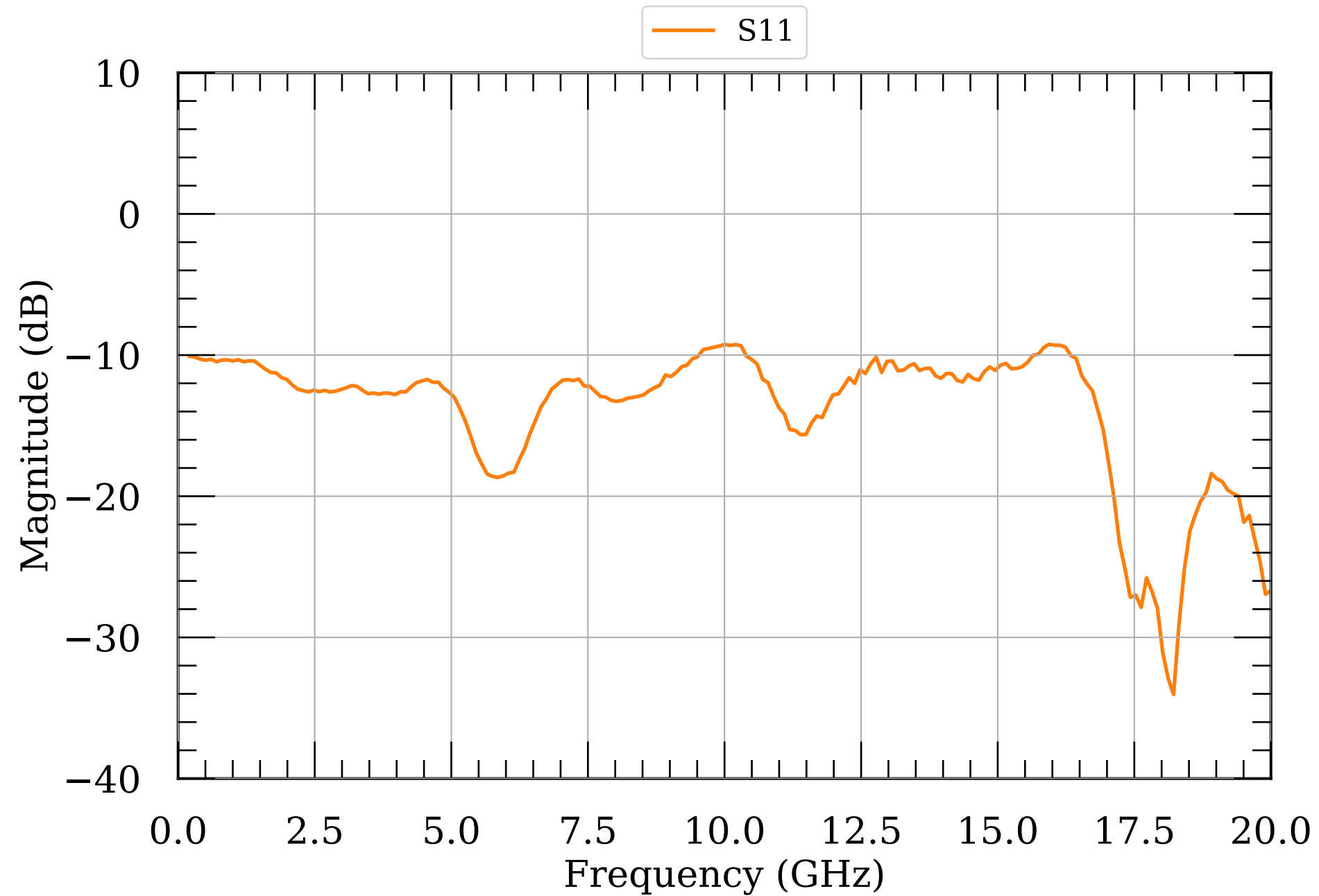
LNA S-params module064v2
